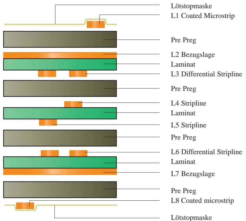
Explosionsansicht eines Testcoupons
