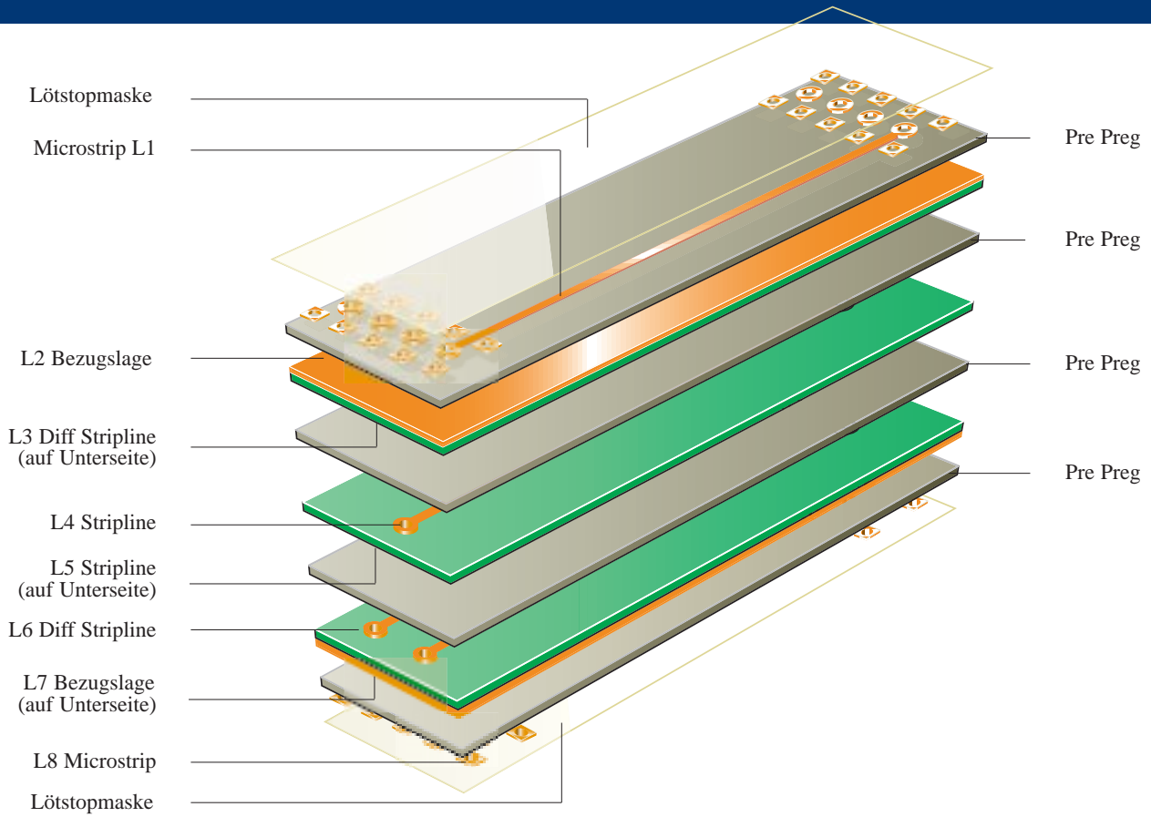
Explosionsansicht eines Testcoupons
